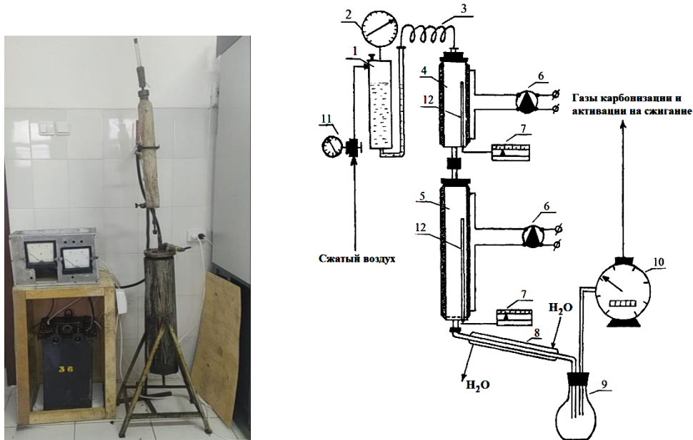
Рисунок. Лабораторная установка получения активированных углей из органического сырья: 1 – емкость для воды; 2 – манометр (образцовый); 3 – медный капилляр; 4 – парогенератор; 5 – печь карбонизации и активации; 6 – латоры; 7 – милливольтметры; 8 – холодильник; 9 – приемник; 10 – газовый счетчик; 11 – стабилизатор давления; 12 – карман термопары
