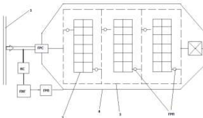
1-рисунок. Трехступенчатая схема газоснабжения населенного пункта: 1 – магистральный газопровод; 2 – газопровод низкого давления; 3 – газопровод среднего давления; 4 – газопровод высокого давления; ГРС – газораспределительная станция;
