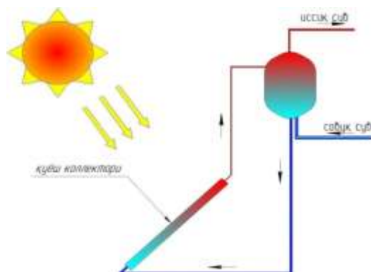
1-rasm. Quyosh kollektorli tabiiy sirkulyatsiyali bir konturli sxema
