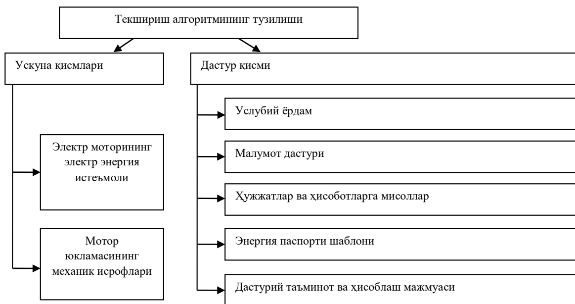
2-расм. Қурилманинг текшириш алгоритми ишлаш структураси.
