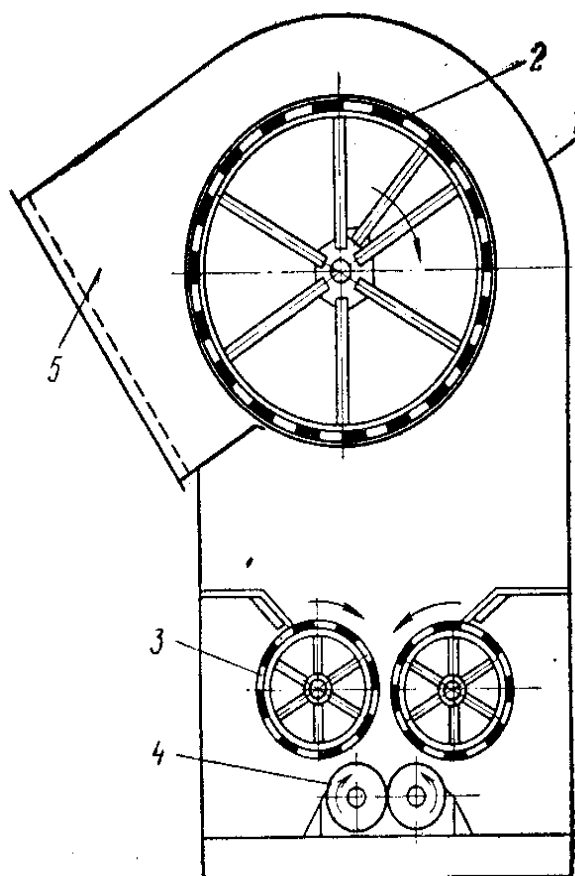
Рис. 1.2. Схема конденсора КВ-3М
