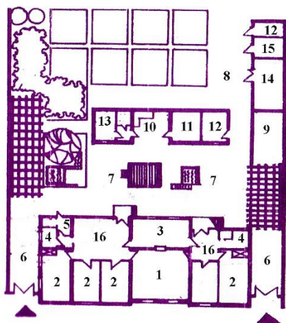
Рис. 2. Жилой дом для сложной семьи: 1 – общая комната; 2 – спальня; 3 – кухня; 4 – ванная; 5 – санузел; 6 – коридор; 7 – жилой дворик; 8 – хозяйственный двор; 9 – гараж; 10 – летняя кухня; 11 – кладовая при кухне; 12 – уборная; 13 – летний душ; 14 – помещения для скота; 15 – помещение для овец; 16 – летнее помещение
