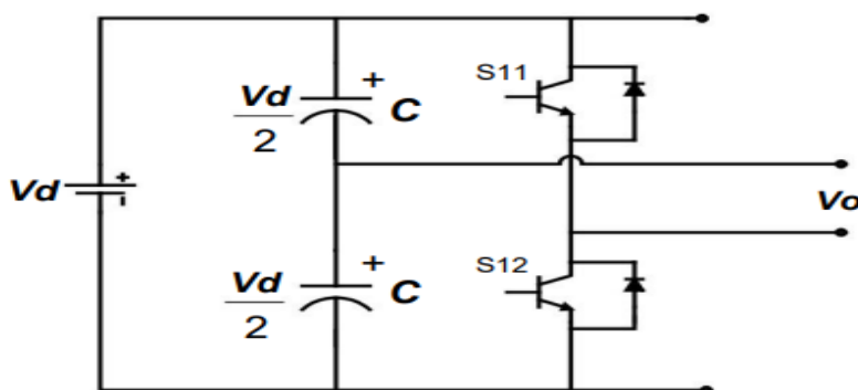
2-rasm. PWM boshqaruv sxemasi.
