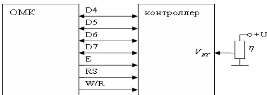
Фигура 2. Программа контроль АСМ под _ связь схема.
