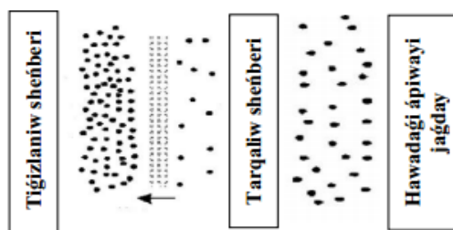
Dene háreketi jónelisi Súwret 1. 5. 2 Dene terbelgende tolqınınıń payda bolıwı
