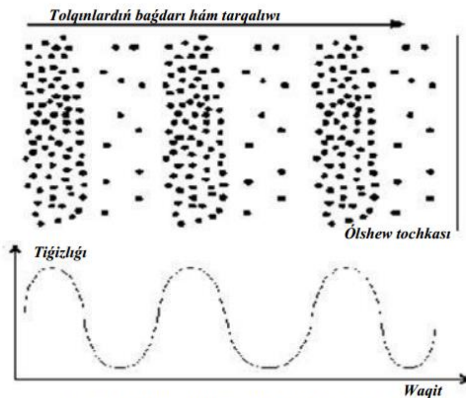
Súwret 1. 5. 3 Hawa tigizlıǵınıń tolqın kóriniside ózgeriwi
